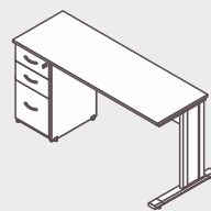
Mesa Diretor Gaveteiro Pedestal 2 gav. Pasta Suspensa Diamante MDGP3G16 L 1,60 | P 0,70 | A 0,75
