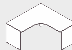
Mesa Estação de trabalho "L" Diamante Pé Painel MLD1212P L 1,20 | P 1,20 | A 0,75 MLD14D13EP L 1,37 | P 1,30 | A 0,75 MLD18D14EP L 1,80 | P 1,37 | A 0,75 MLD13E12DP L 1,30 | P 1,20 | A 0,75 MLD15E13DP L 1,50 | P 1,30 | A 0,75 MLD1515P L 1,50 | P 1,50 | A 0,75 MLD13D12EP L 1,30 | P 1,20 | A 0,75 MLD15D13EP L 1,50 | P 1,30 | A 0,75 MLD16E15DP L 1,60 | P 1,50 | A 0,75 MLD14E12DP L 1,37 | P 1,20 | A 0,75 MLD16E13DP L 1,60 | P 1,30 | A 0,75 MLD16D15EP L 1,60 | P 1,50 | A 0,75 MLD14D12EP L 1,37 | P 1,20 | A 0,75 MLD16D13EP L 1,60 | P 1,30 | A 0,75 MLD18E15DP L 1,80 | P 1,50 | A 0,75 MLD15E12DP L 1,50 | P 1,20 | A 0,75 MLD18E13DP L 1,80 | P 1,30 | A 0,75 MLD18D15EP L 1,80 | P 1,50 | A 0,75 MLD15D12EP L 1,50 | P 1,20 | A 0,75 MLD18D13EP L 1,80 | P 1,30 | A 0,75 MLD1616P L 1,60 | P 1,60 | A 0,75 MLD16E12DP L 1,60 | P 1,20 | A 0,75 MLD1414P L 1,37 | P 1,37 | A 0,74 MLD18E16DP L 1,80 | P 1,60 | A 0,75 MLD16D12EP L 1,60 | P 1,20 | A 0,75 MLD15E14DP L 1,50 | P 1,37 | A 0,75 MLD18D16EP L 1,80 | P 1,60 | A 0,75 MLD18D12EP L 1,80 | P 1,20 | A 0,75 MLD15D14EP L 1,50 | P 1,37 | A 0,75 MLD1818P L 1,80 | P 1,80 | A 0,75 MLD1313P L 1,30 | P 1,30 | A 0,75 MLD16E14DP L 1,60 | P 1,37 | A 0,75 MLD14E13DP L 1,37 | P 1,30 | A 0,75 MLD16D14EP L 1,60 | P 1,37 | A 0,75 MLD18E14DP L 1,80 | P 1,37 | A 0,75
