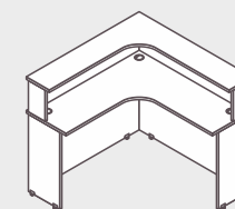
Balcão de Atendimento Plus BAS12 L 1,20 | P 1,20 | A 1,10 BAS14 L 1,37 | P 1,37 | A 1,10
