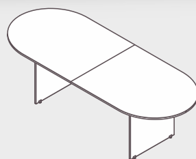
Mesa Reunião Oval Diamante Pé Painel MRVD35P L 3,50 | P 1,00 | A 0,75
