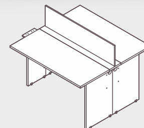
Mesa Plataforma Fim Passa Fio Diamante MPDF12P L 1,20 | P 1,20 | A 0,75
