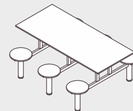
Refeitório Banco Redondo Plus RBR510 L 2,70 | P 1,40 | A 0,75 RBR58 L 2,40 | P 1,40 | A 0,75 RBR56 L 1,80 | P 1,40 | A 0,75 RBR54 L 1,20 | P 1,40 | A 0,75
