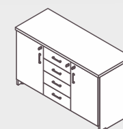
Credenza 4 Gavetas Safira CRF6 L 1,29 | P 0,41 | A 0,75 Corrediça Telescópica
