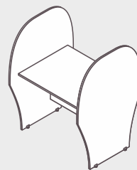
Cabine de Atendimento Completa Plus CATS84 L 0,83 | P 1,15 | A 1,26 CATS100 L 0,98 | P 1,15 | A 1,26 CATS124 L 1,23 | P 1,15 | A 1,26
