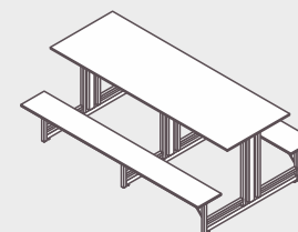
Refeitório Completo Plus RCS10 L 2,70 | P 1,40 | A 0,75 RCS8 L 2,40 | P 1,40 | A 0,75 RCS6 L 1,80 | P 1,40 | A 0,75 RCS4 L 1,20 | P 1,40 | A 0,75
