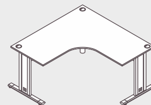
Mesa Estação de trabalho "L" Diamante MLD1212 L 1,20 | P 1,20 | A 0,75 MLD1414 L 1,37 | P 1,37 | A 0,75 MLD1213 L 1,20 | P 1,30 | A 0,75 MLD1415 L 1,37 | P 1,50 | A 0,75 MLD1214 L 1,20 | P 1,37 | A 0,75 MLD1416 L 1,37 | P 1,60 | A 0,75 MLD1215 L 1,20 | P 1,50 | A 0,75 MLD1418 L 1,37 | P 1,80 | A 0,75 MLD1216 L 1,20 | P 1,60 | A 0,75 MLD1515 L 1,50 | P 1,50 | A 0,75 MLD1218 L 1,20 | P 1,80 | A 0,75 MLD1518 L 1,50 | P 1,80 | A 0,75 MLD1313 L 1,30 | P 1,30 | A 0,75 MLD1516 L 1,50 | P 1,60 | A 0,75 MLD1314 L 1,30 | P 1,37 | A 0,75 MLD1616 L 1,60 | P 1,60 | A 0,75 MLD1315 L 1,30 | P 1,50 | A 0,75 MLD1618 L 1,60 | P 1,80 | A 0,75 MLD1316 L 1,30 | P 1,60 | A 0,75 MLD1818 L 1,80 | P 1,80 | A 0,75 MLD1318 L 1,30 | P 1,80 | A 0,75
