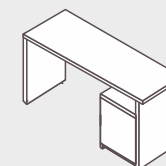
Mesa Essencial Diamante MESD L 1,20 | P 0,45 | A 0,75
