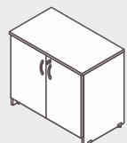
Armário Secretária Plus ASS2 L 0,91 | P 0,41 | A 0,75 ASS2P46 L 0,91 | P 0,46 | A 0,75
